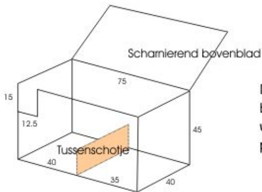
Schema van een broedkast voor de kerkuil (oud hout gebruiken), maten in cm.
